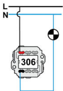
Interrupor Switch Interrupteur
