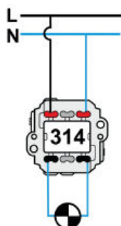
Interrupor bipolar Double pole switch Interrupteur bipolaire
