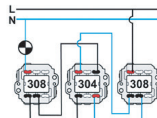
Cruzamiento Intermediate switch Permutateur
