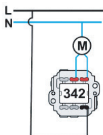
Interruptor de persianas Switch for blinds Interrupteur pour volets roulants
