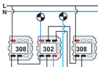
Doble conmutador Double two-way switch Double va-et-vient
