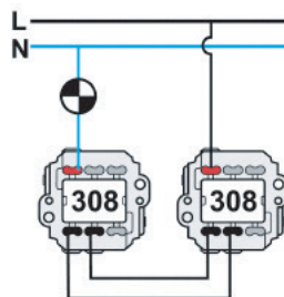
Conmutador Two-way switch Va-et-vient
