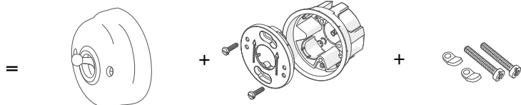
Mecanismo Dimbler sin paso de cable (pág. 63)
